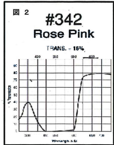
透過率特性データグラフ見本
